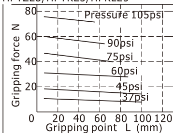
HFTZ25/HFTK25/HFKL25
