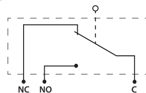
NVS 5 - Styk przełączny
