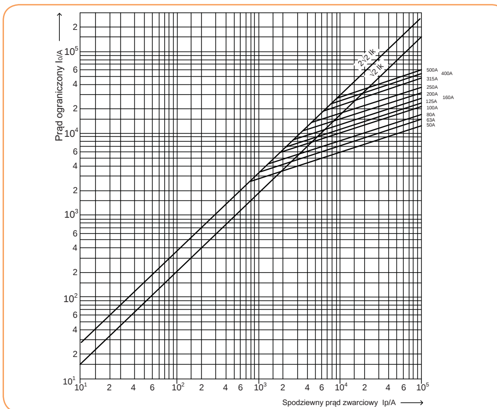
Charakterystyki prądów ograniczonych wkładek topikowych o charakterystyce gG - 1200V - 1XL, 2XL, 3L
