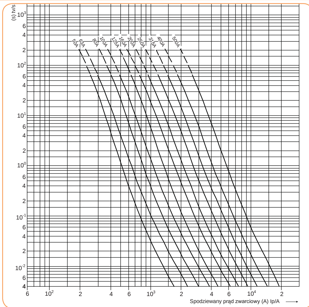
Charakterystyki czasowo - prądowe (rzeczywiste) wkładek topikowych o charakterystyce gG - 1200V - 1XL, 2XL, 3L
