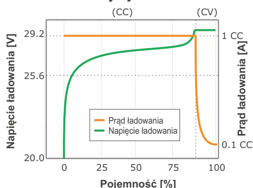
Charakterystyka ładowania
