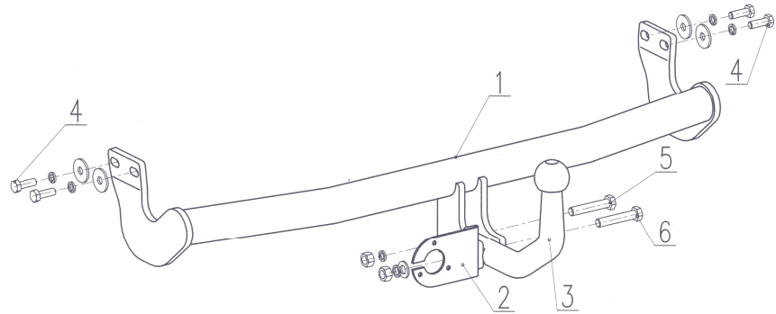
Bild 2.: Ausschnitt der Heckstosstange
