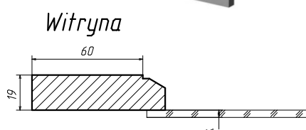
Witryna podfrezowanie
