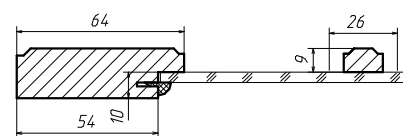
Szpros podfrezowanie
