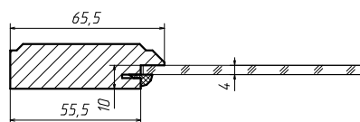
Witryna podfrezowanie
