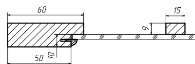
Szpros podfrezowanie
