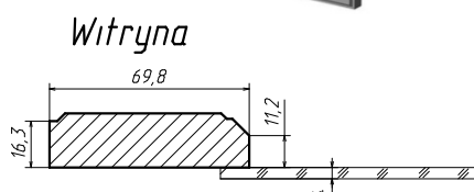
Witryna podfrezowanie
