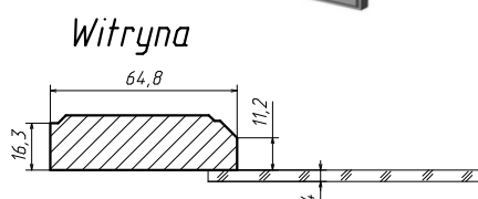
Witryna podfrezowanie
