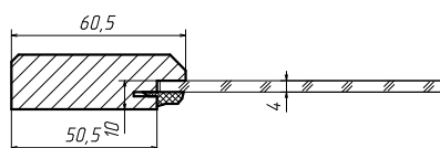
Witryna podfrezowanie
