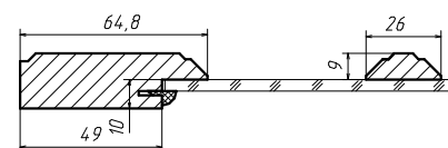
Szpros podfrezowanie
