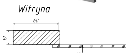
Witryna podfrezowanie
