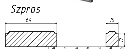
Szpros podfrezowanie
