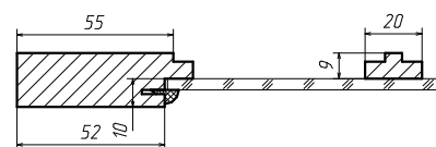
Szpros podfrezowanie
