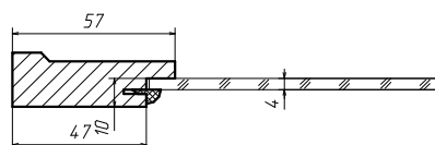
Witryna podfrezowanie
