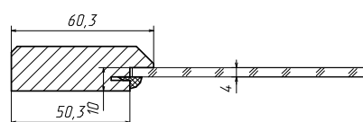
Witryna podfrezowanie
