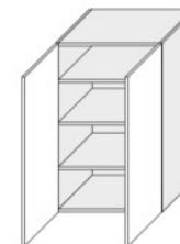
W4 60 2F (600/960/325)
