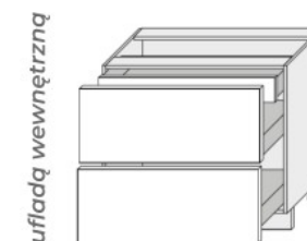
D2A/90/1A (900/820/500)
