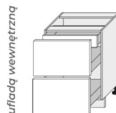
D2A/60/1A (600/820/500)
