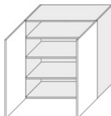
W4 90 (900/960/325)
