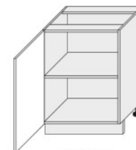
D1D 60 (600/820/500)
