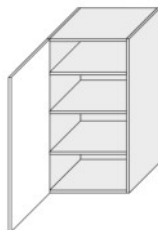
W4 45 (450/960/325)
