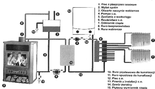
Schemat podłączenia pieca z płaszczem wodnym z kotłem gazowym
