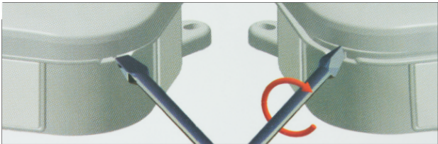
Rys. 1.: Sposób otwierania pokrywy typu "klik"
