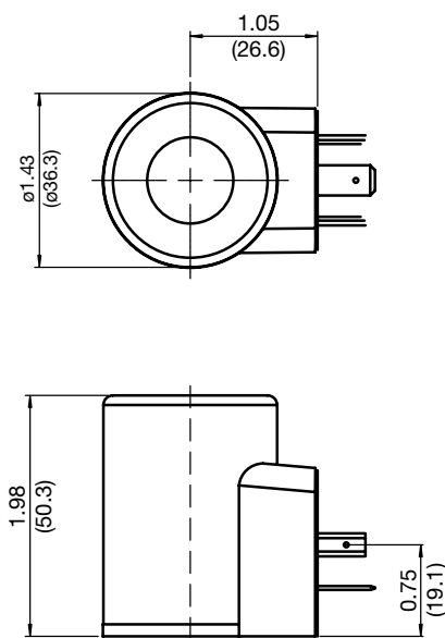
Din 175301
