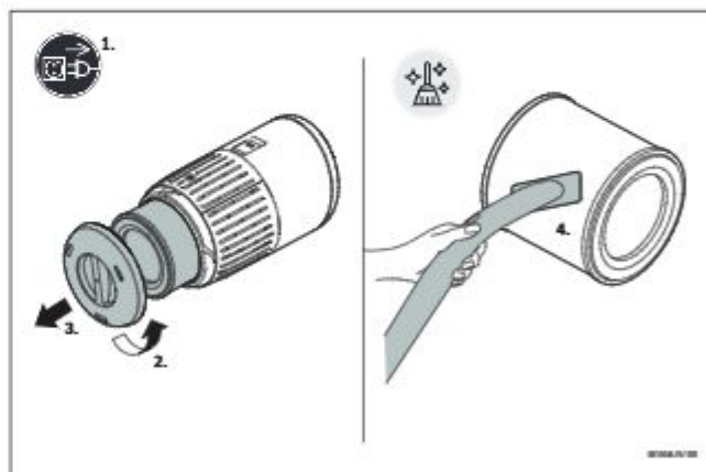
Fig. 106 Rimozione e pulizia del filtro
