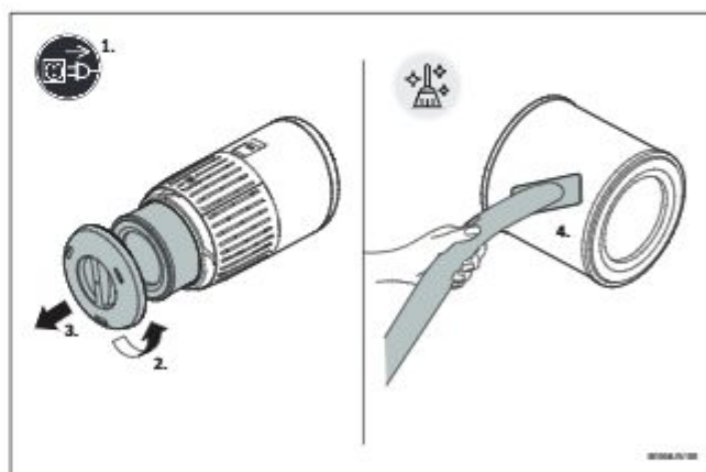
Fig. 34 Afmontering og rengøring af filteret
