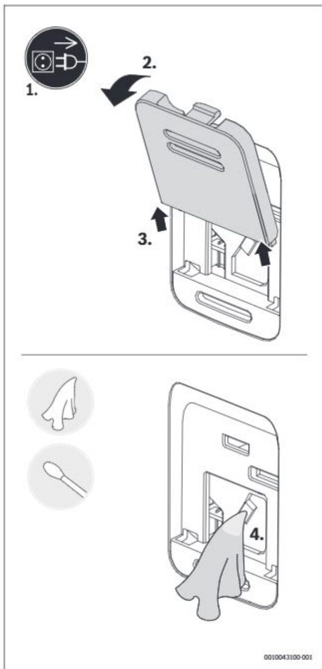
Afb. 117 Reinigen van de luchtkwaliteitsensor
