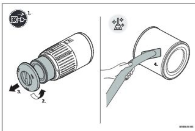
Bild 46 Abnehmen und Reinigen des Filters
