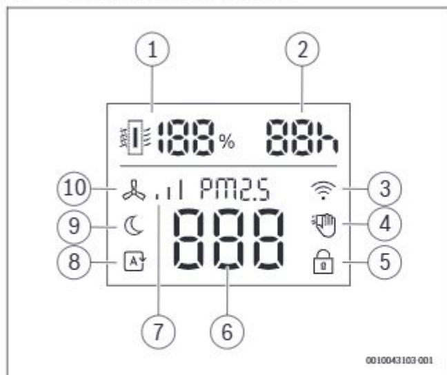
Bild 40 Übersicht Benutzerschnittstelle
