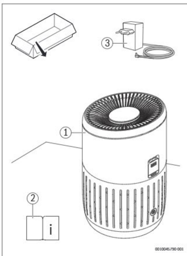
Afb. 109 Leveringsomvang
