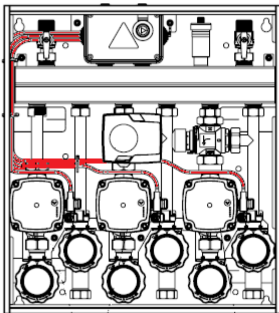
Rysunek 13: Fabryczne rozprorowadzenie przewodów elektrycznych
