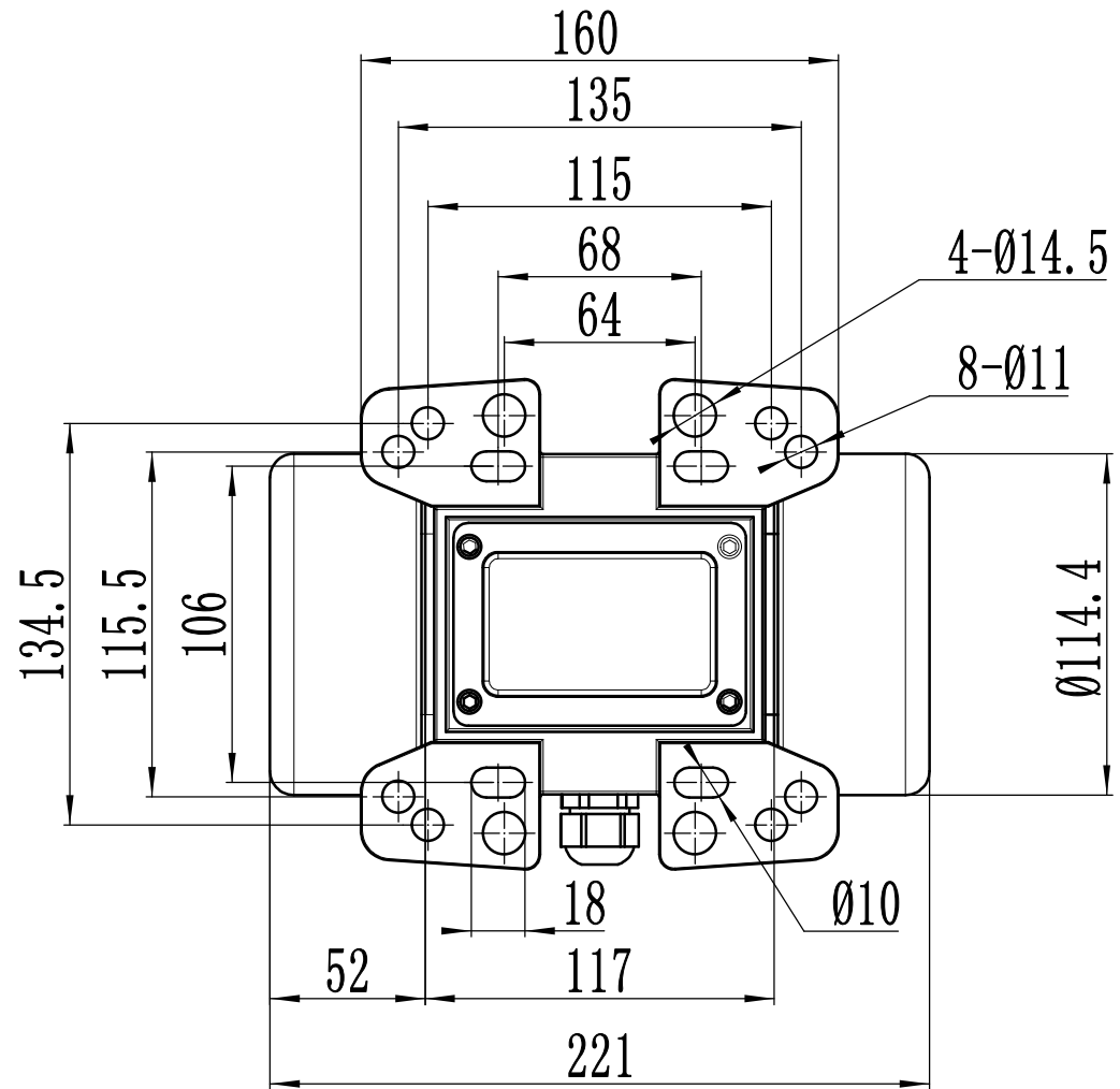
机座23 (Frame 23)
