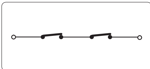
Rys. Połączenie szeregowe 2 styków N.C.
