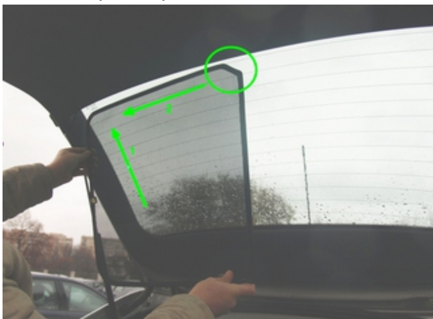
Rys.5 - Montaż zasłonek klapy bagażnika
