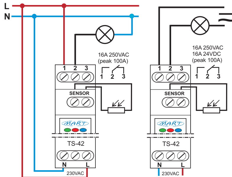
Rys 2. Schematy podłączenia AUTOMATU ZMIERZCHOWEGO TS-42-4.
