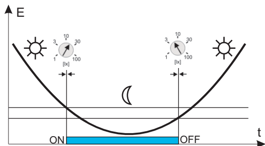
Rys 3. Schemat poglądowy zasady działania AUTOMATU ZMIERZCHOWEGO TS-42-4.
