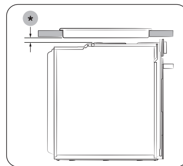
Instalacja z płytą grzejną
