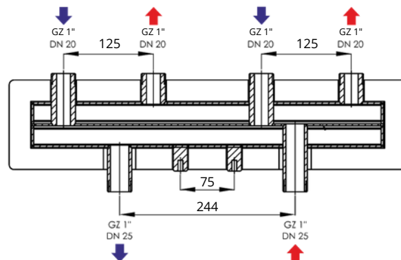
2 obiegi DN20 GZ
