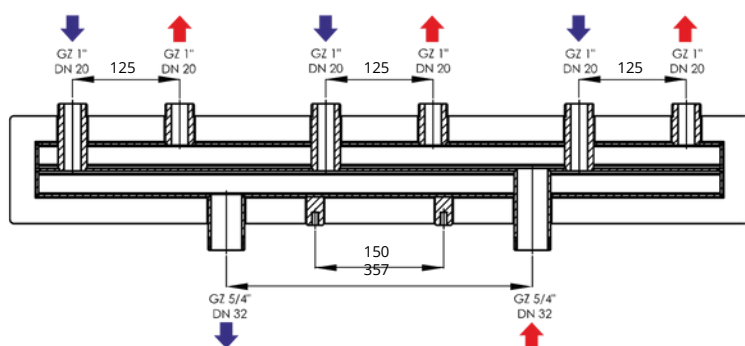
3 obiegi DN20 GZ
