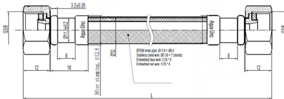
Wężyk przyłączeniowy 3/8" x 3/8"
