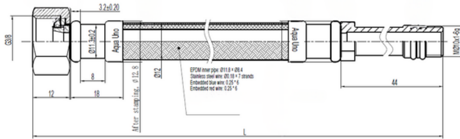
Wężyk przyłączeniowy do baterii G3/8 x M10
