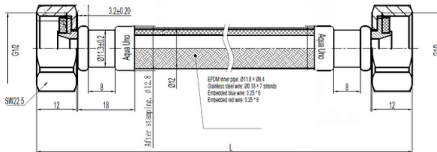
Wężyk przyłączeniowy 1/2" x 1/2"
