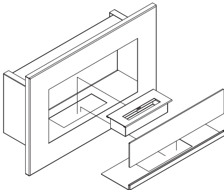
Rys. 7. Montaż szyby wraz z dedykowaną podstawą na przykładzie biokominka Delta
