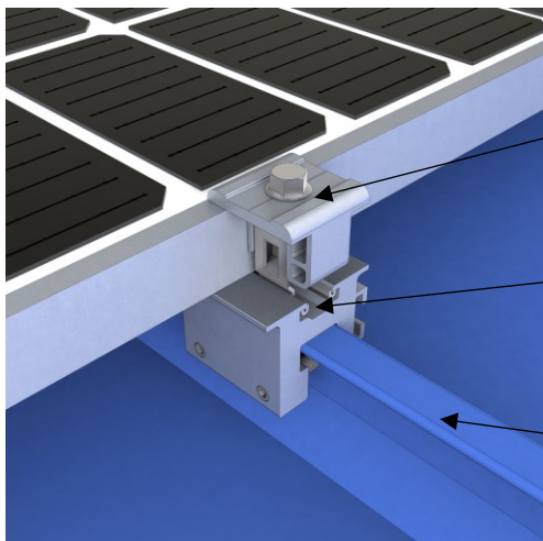
Abrazadera universal (NXT-AU) en modo de remate
