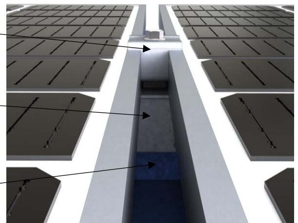
Abrazadera universal (NXT-AU) en modo intermedio
