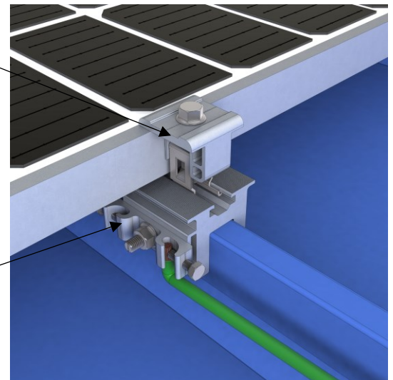
Instalación de terminal de tierra (NXT-GC)
