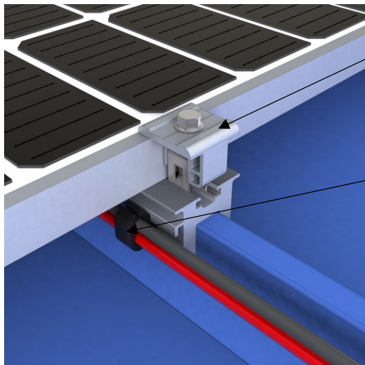
Instalación de clip de plástico para cables (NXT-CLIP)
