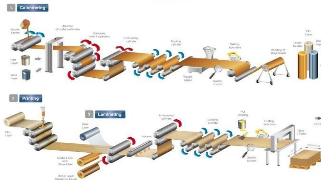
Figure 1 : Procédé de fabrication des produits LVT Glue down
