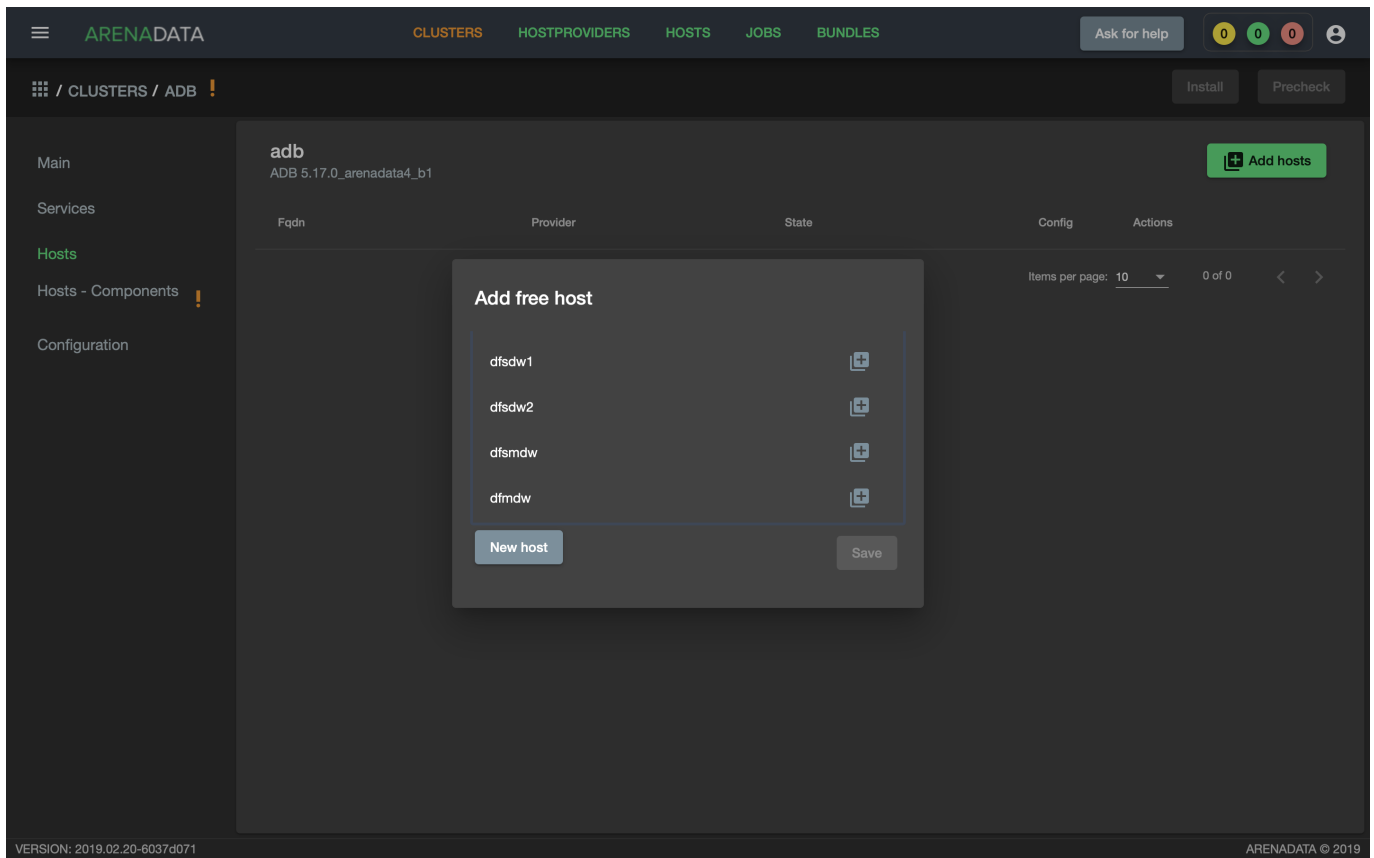
Рис.3.18.: Выбор хостов
