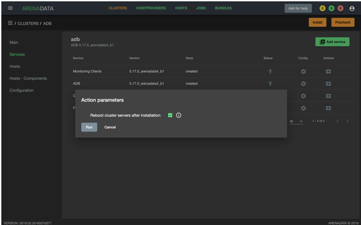
Рис.3.34.: Action parameters
