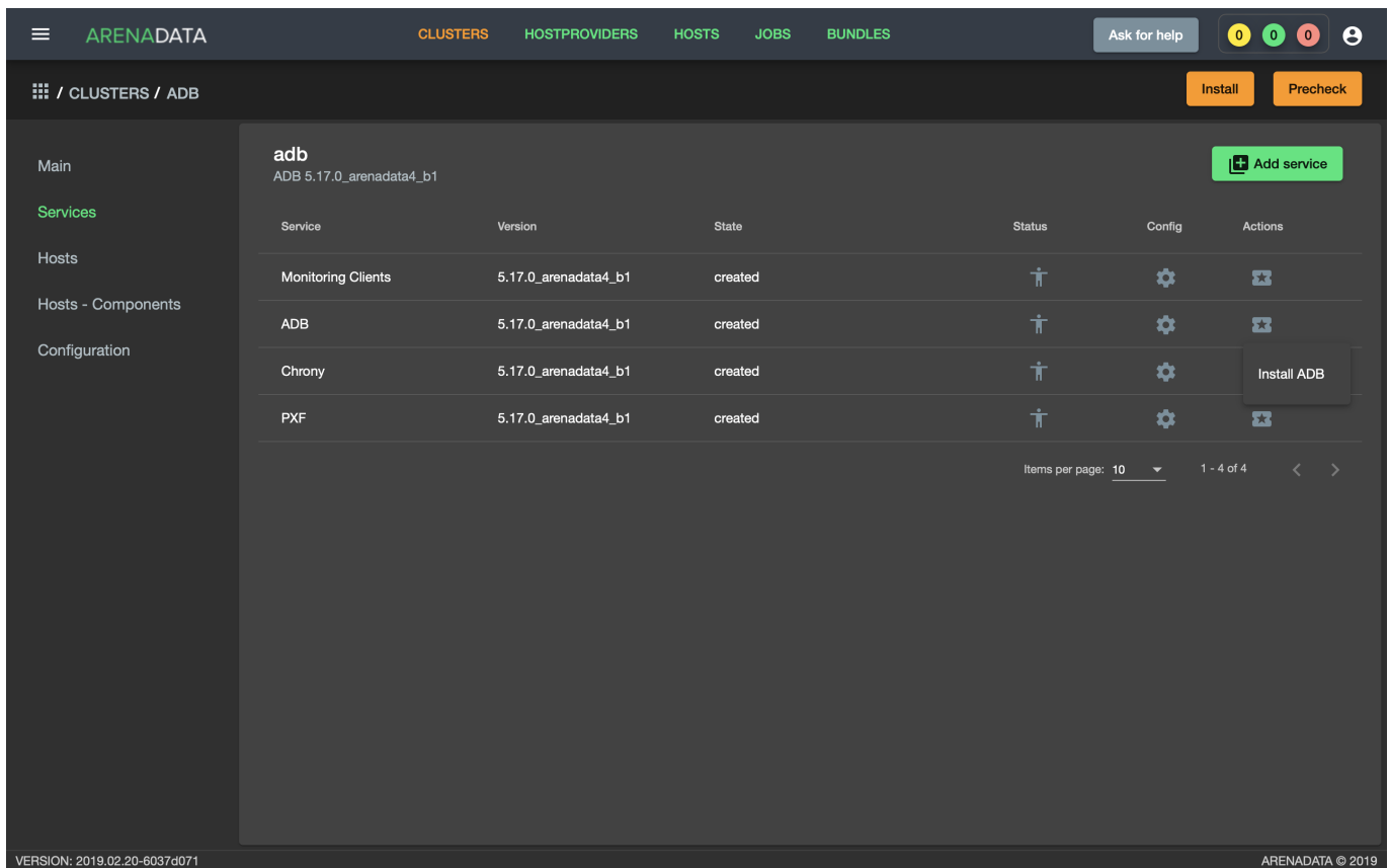
Рис.3.33.: Install ADB
