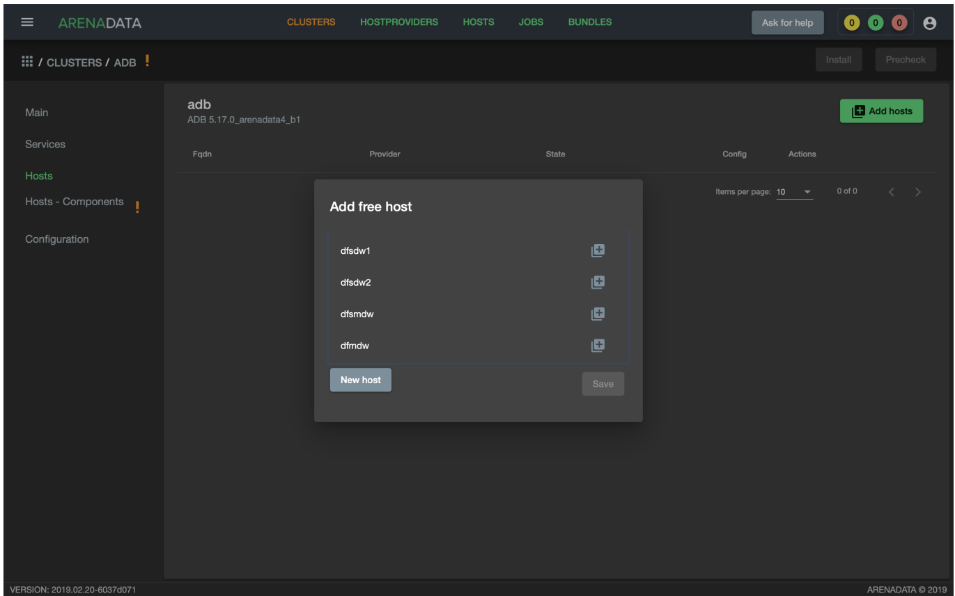
Рис.3.18.: Выбор хостов
