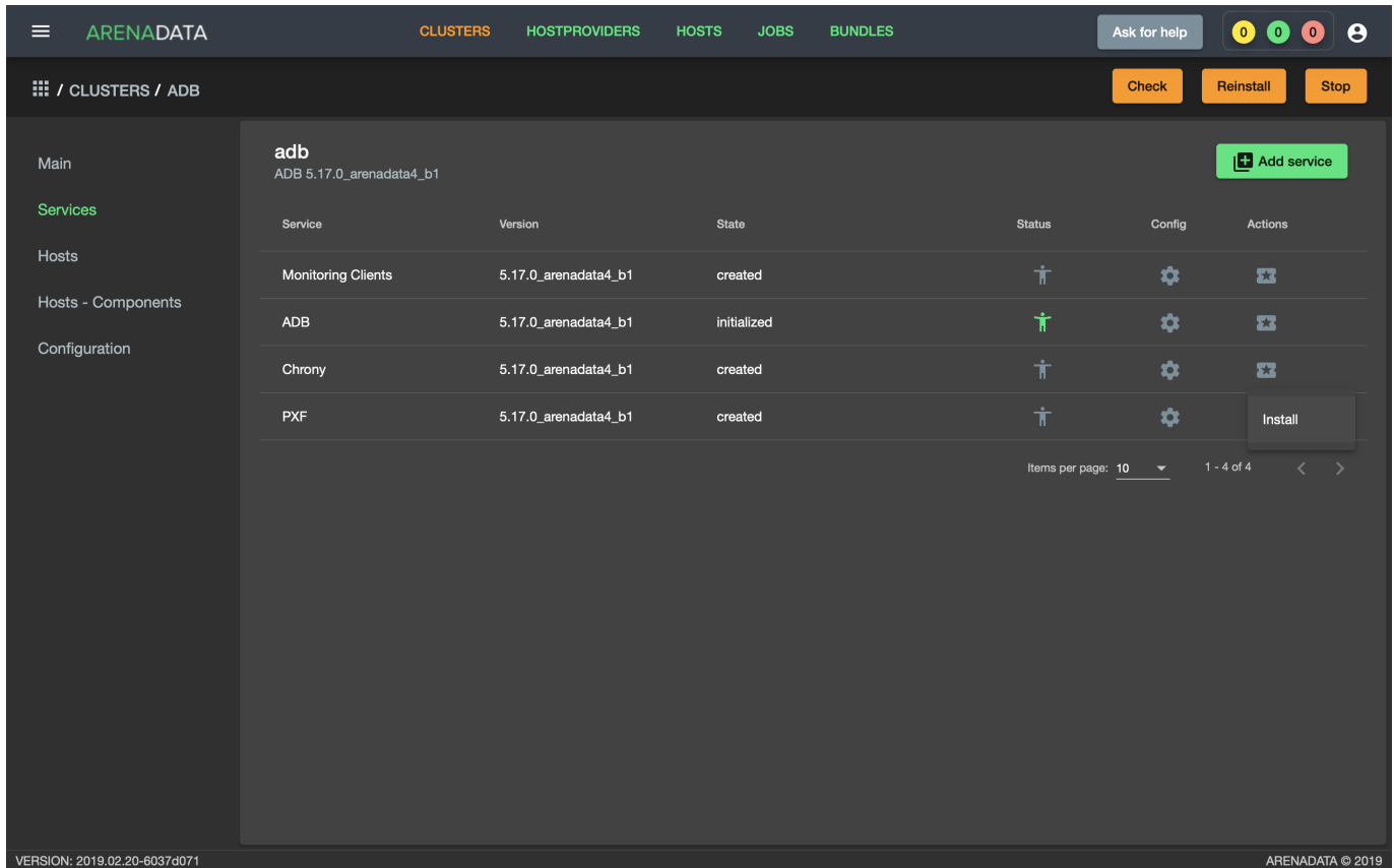
Рис.3.41.: Install Chrony
