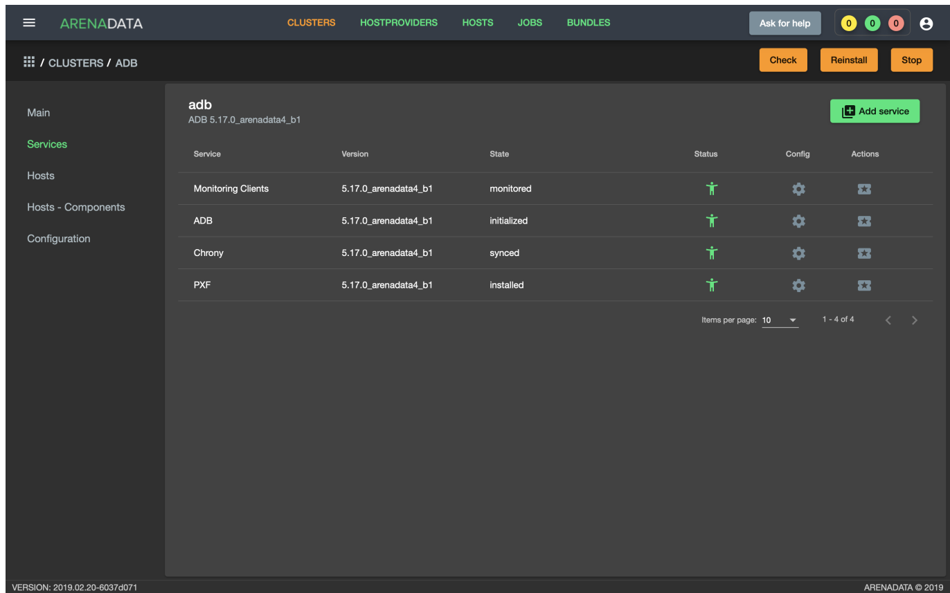
Рис.3.32.: Статус сервисов
