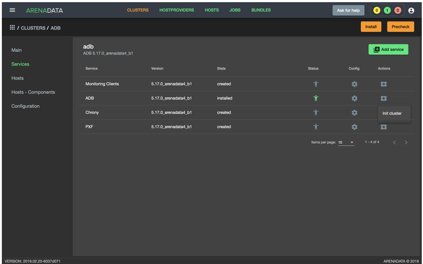
Рис.3.36.: Init cluster
