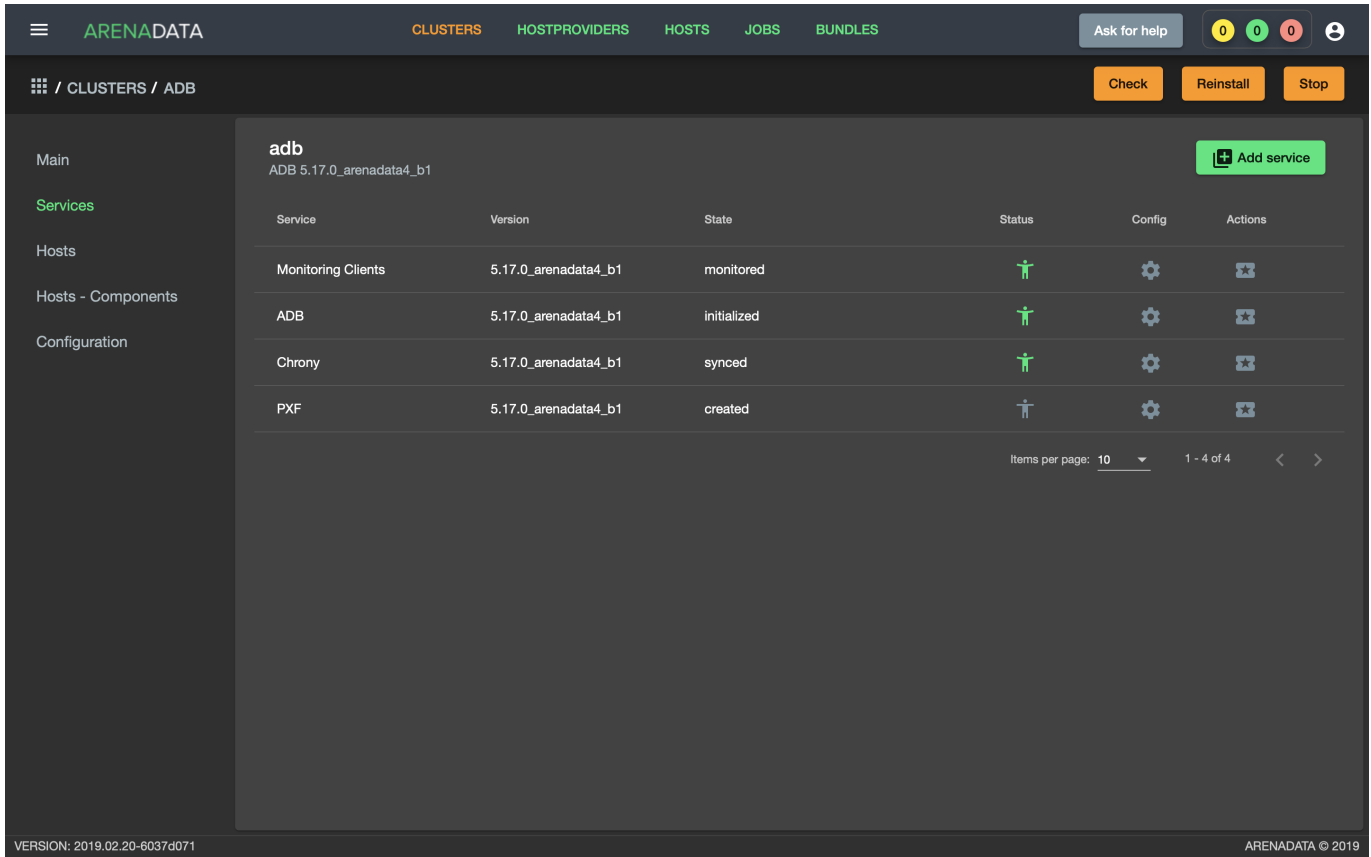
Рис.3.46.: Статус сервиса
