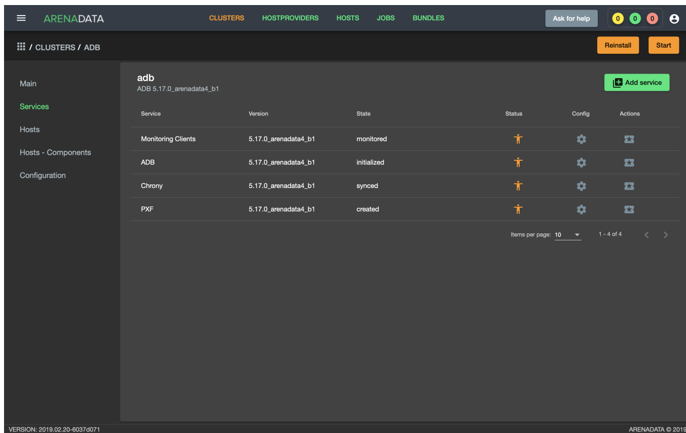
Рис.4.7.: Статусы сервисов
