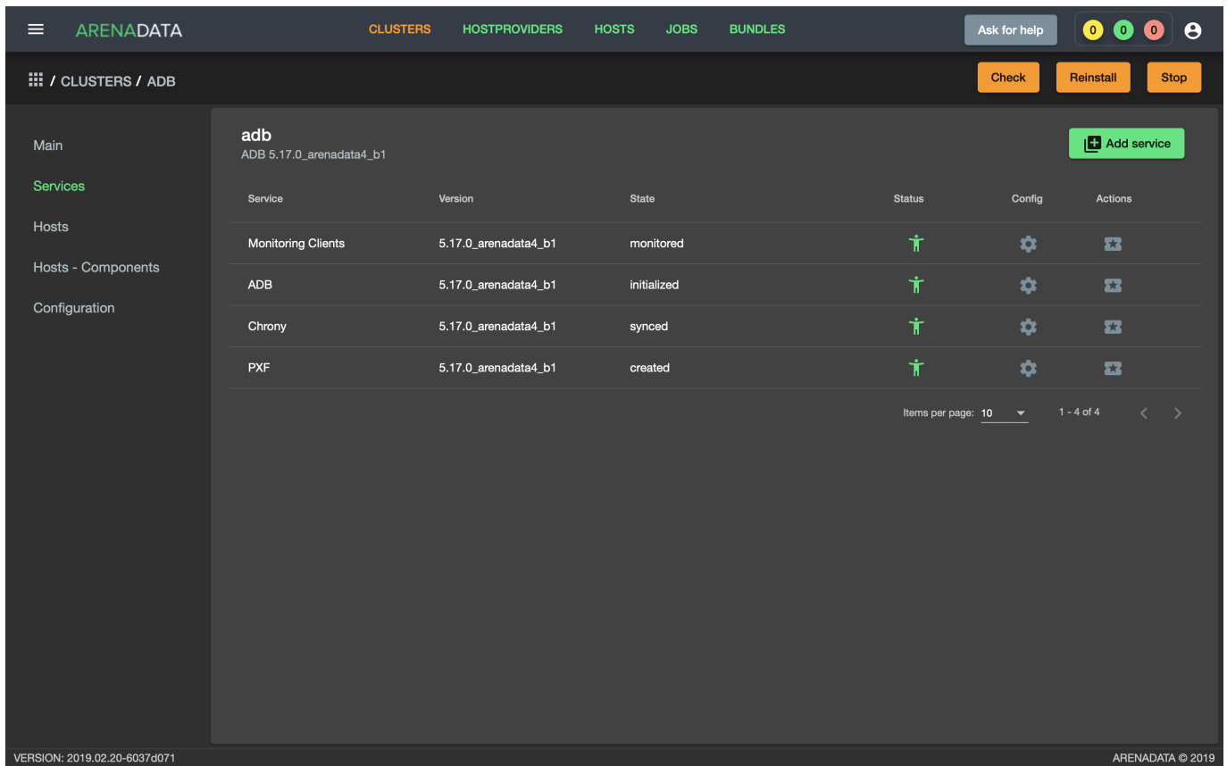
Рис.4.5.: Остановка кластера
