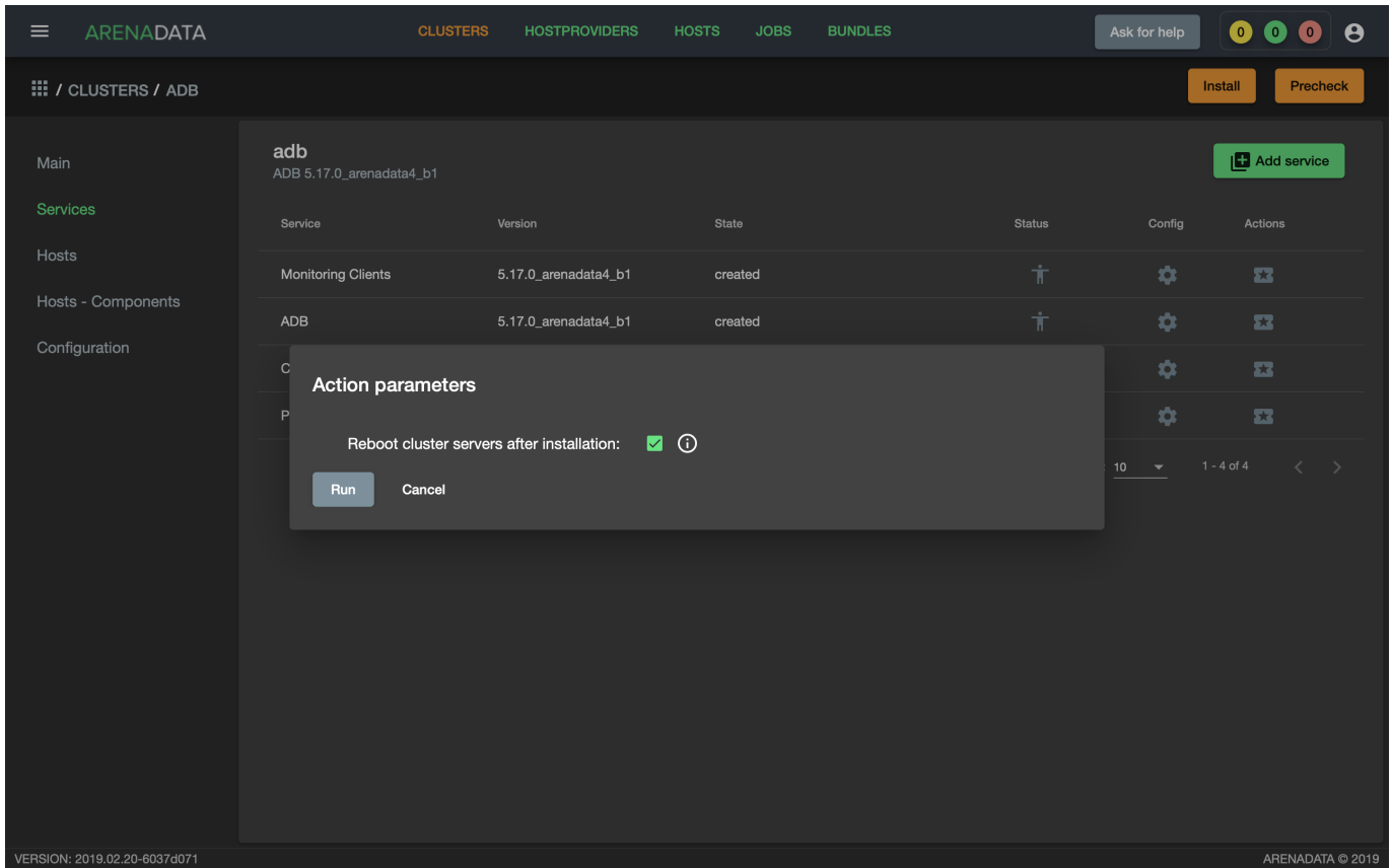
Рис.3.34.: Action parameters
