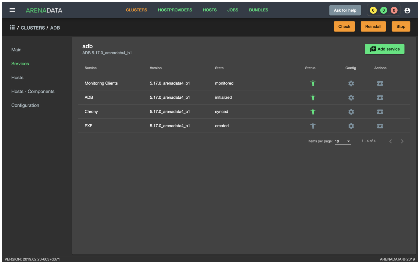
Рис.3.46.: Статус сервиса
