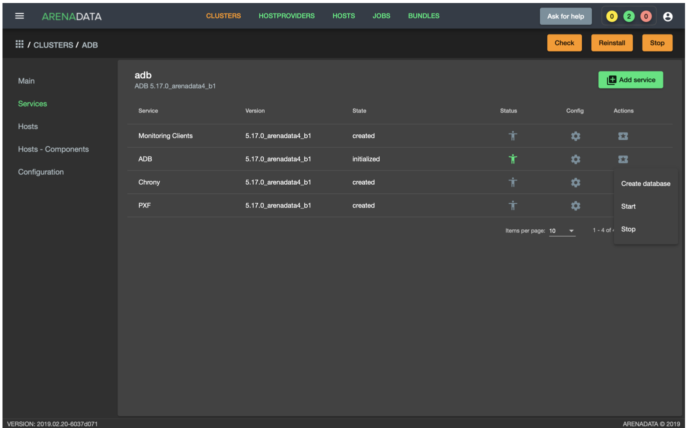
Рис.3.40.: Create database
