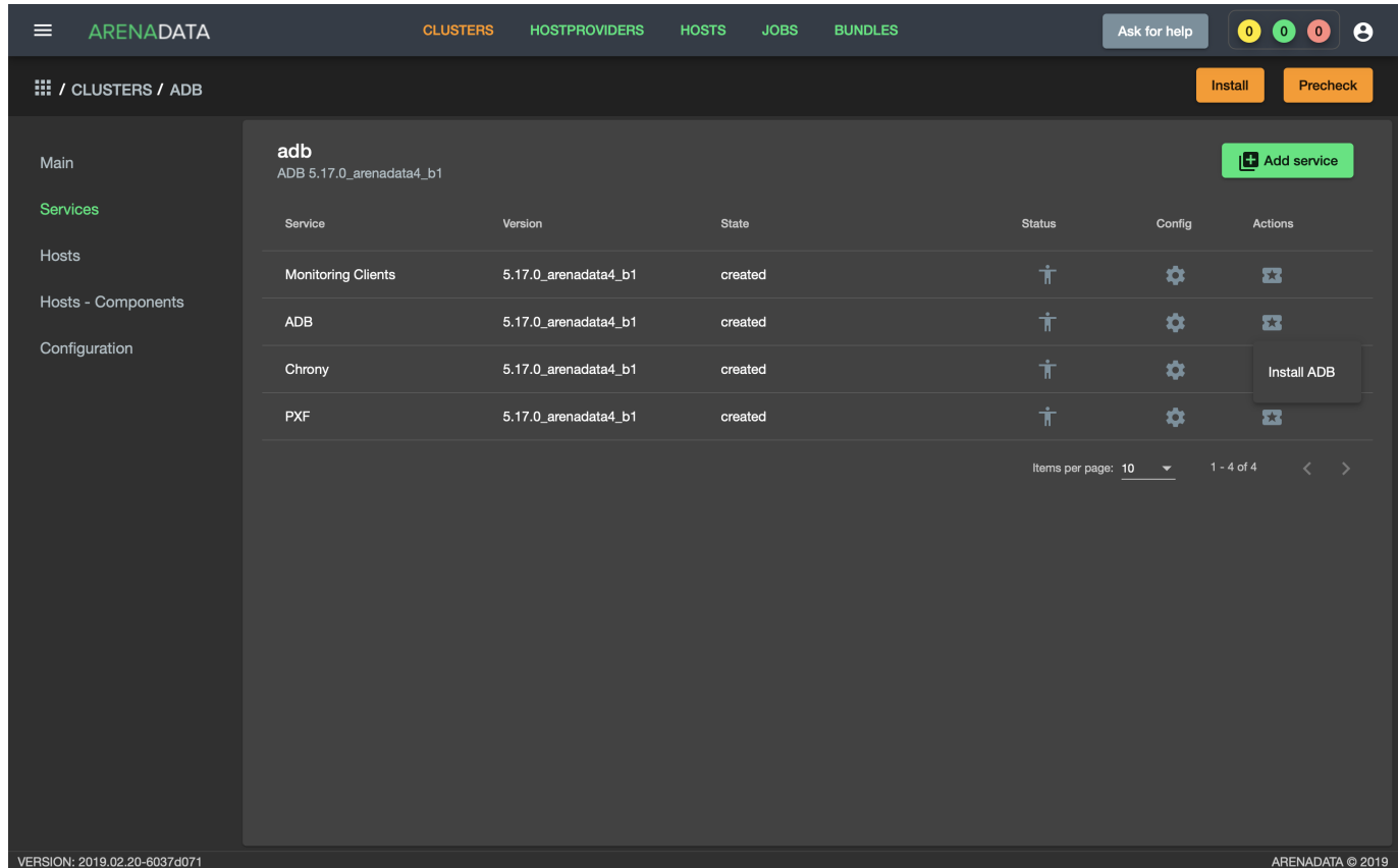
Рис.3.34.: Install ADB
