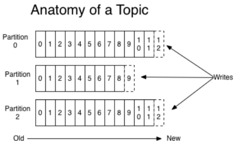
Рис.1.1.: Партиционированный журнал
