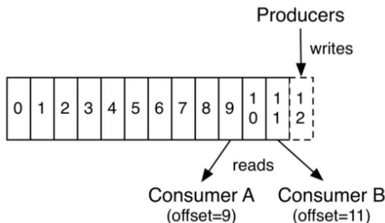
Рис.1.2.: Логика смещения
