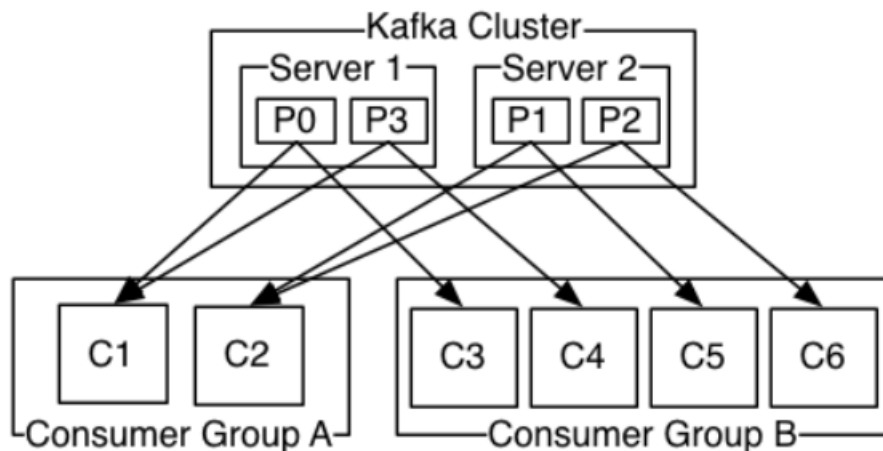
Рис.1.3.: Группы потребителей
