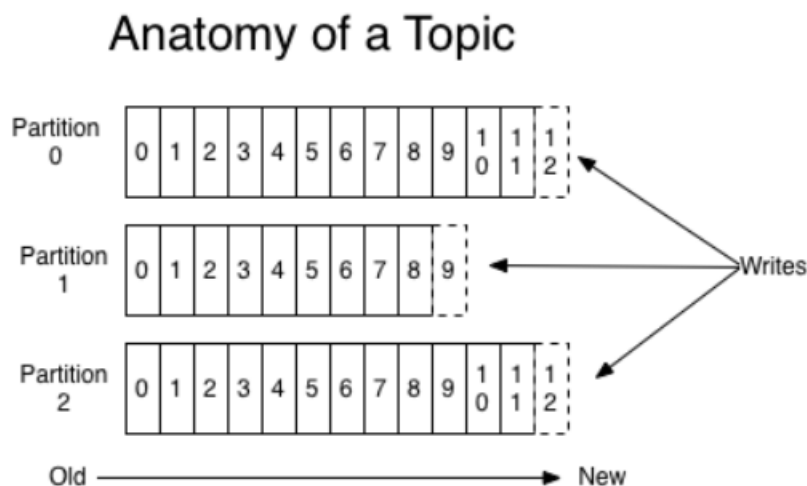
Рис.1.1.: Партиционированный журнал
