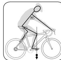
Le genou doit se trouver à la verticale de l'axe de la pédale avant
