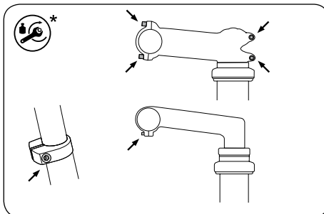
Mögliche Positionen von Schraubverbindungen zur Anpassung
