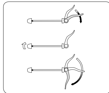
Einstellmutter lockern
