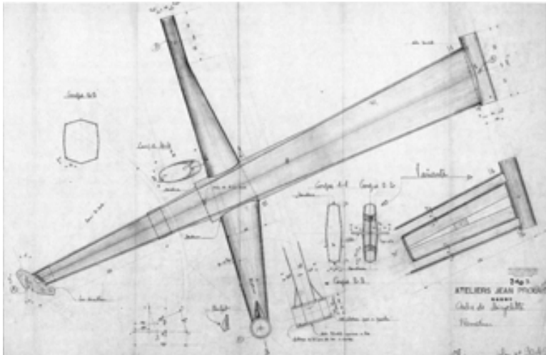
plan d'exécution du cadre de bicyclette par Jean Prouvé
