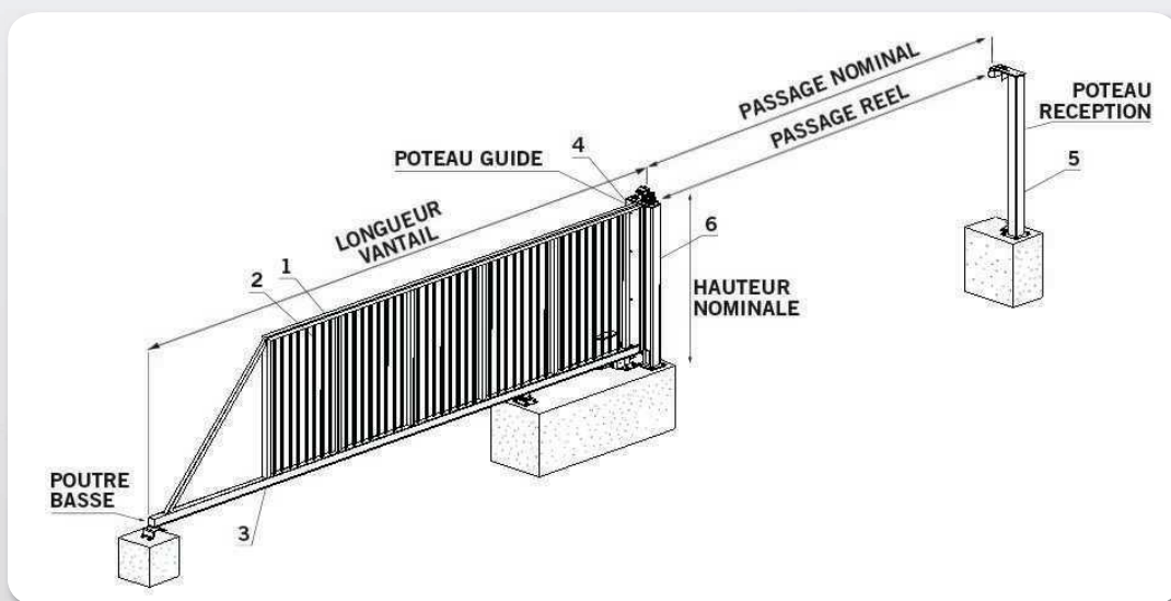
Poutre 150x120 mm (modèle B) pour les passages de 6,5 m à 8 m
