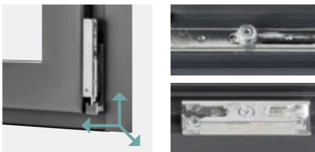
Réglage tri-dimensionnel du palier d'angle : réglage latéral, en hauteur et en compression
