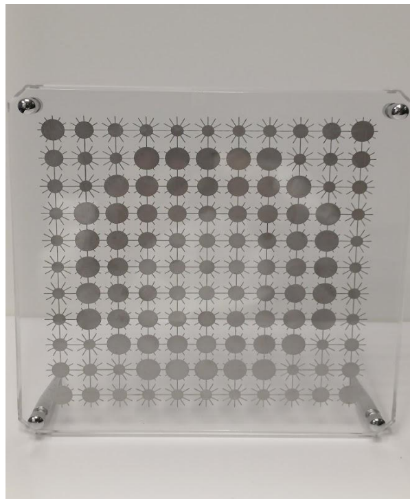
X Band 天線 (X Band Antenna)
