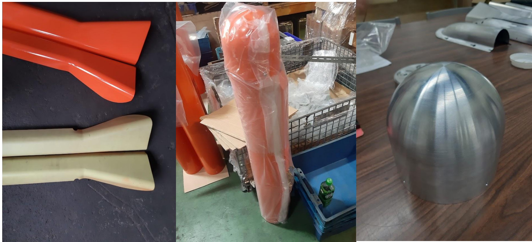
無人機金屬件系列 (Drone Metal Parts)
