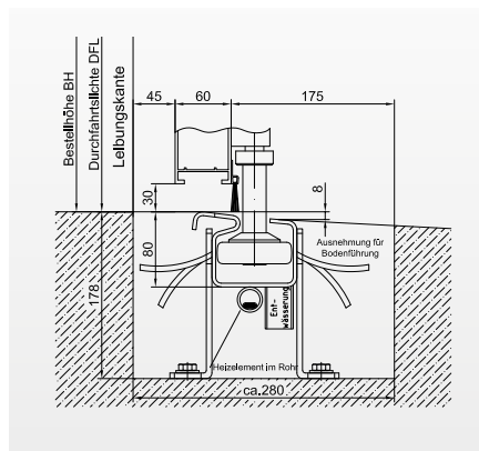
Bodenführung
