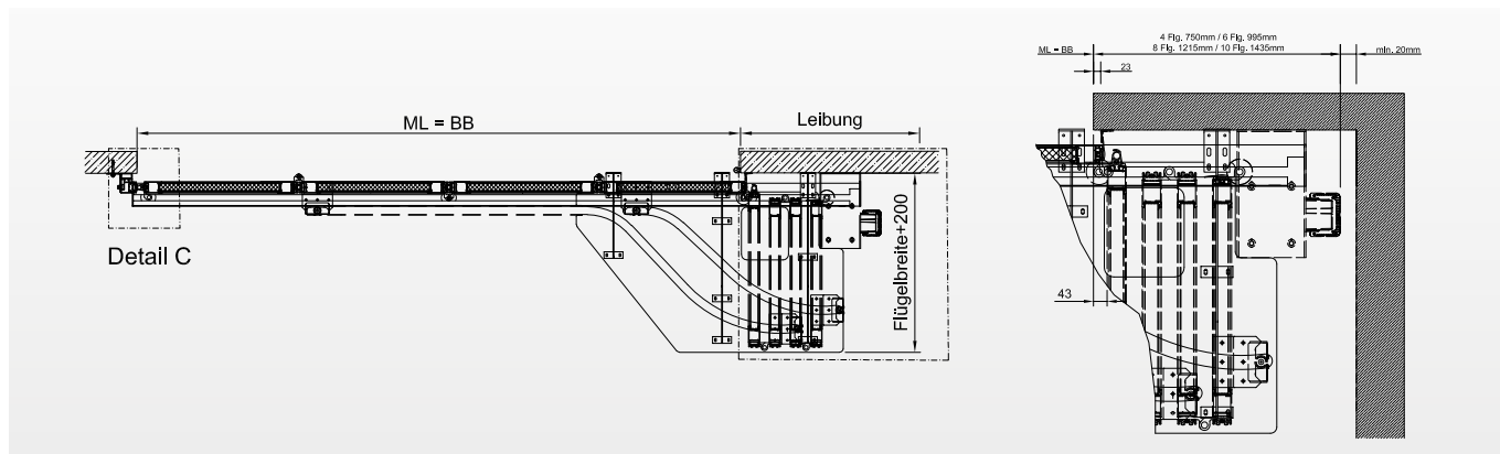
Horizontalschnitt
