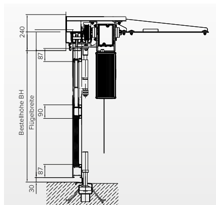
Vertikalschnitt
