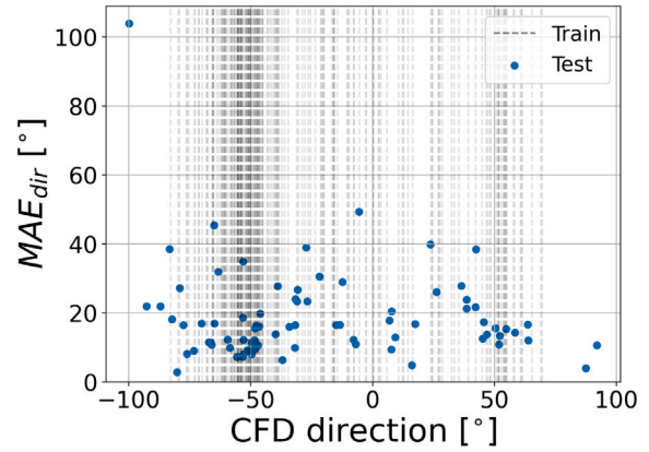
(d) MAE_{dir} versus CFD wind direction.
