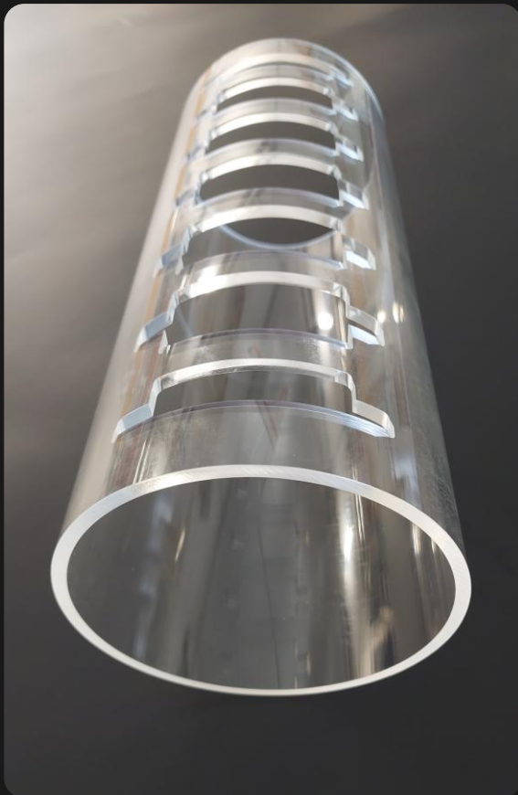
PC – késvédő burkolat/élelmiszeripari gép
