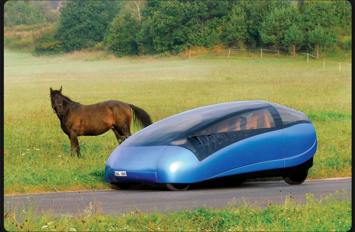
PMMA GS – hőformázott járműburkolati elemek és ablakok
