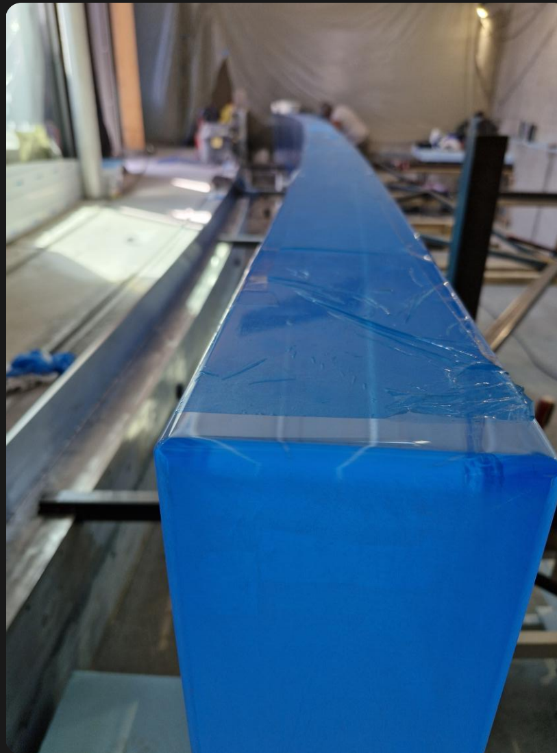
150 mm PMMA GS – hőformázott, polírozott és ragasztott medencefal
