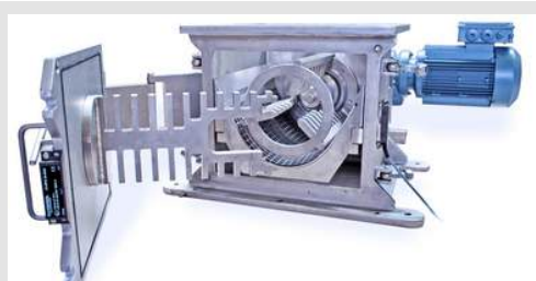
KLONTENBREKERS
