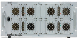
ZTM2-1 8 x SP4T (18 GHz) 4 x SPDT (18 GHz)
