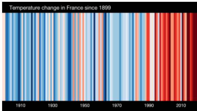
Réchauffement climatique
