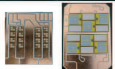
GaN 1µm BONDLINE & DOBLE SIDE COOLING
