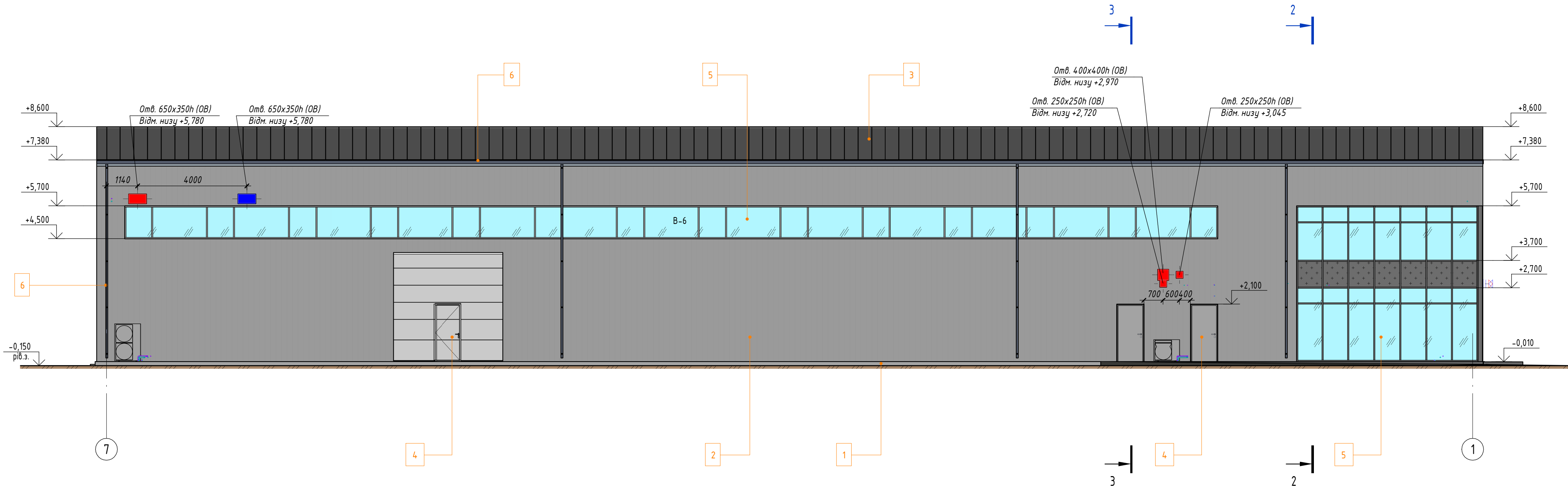
Фасад К - А
