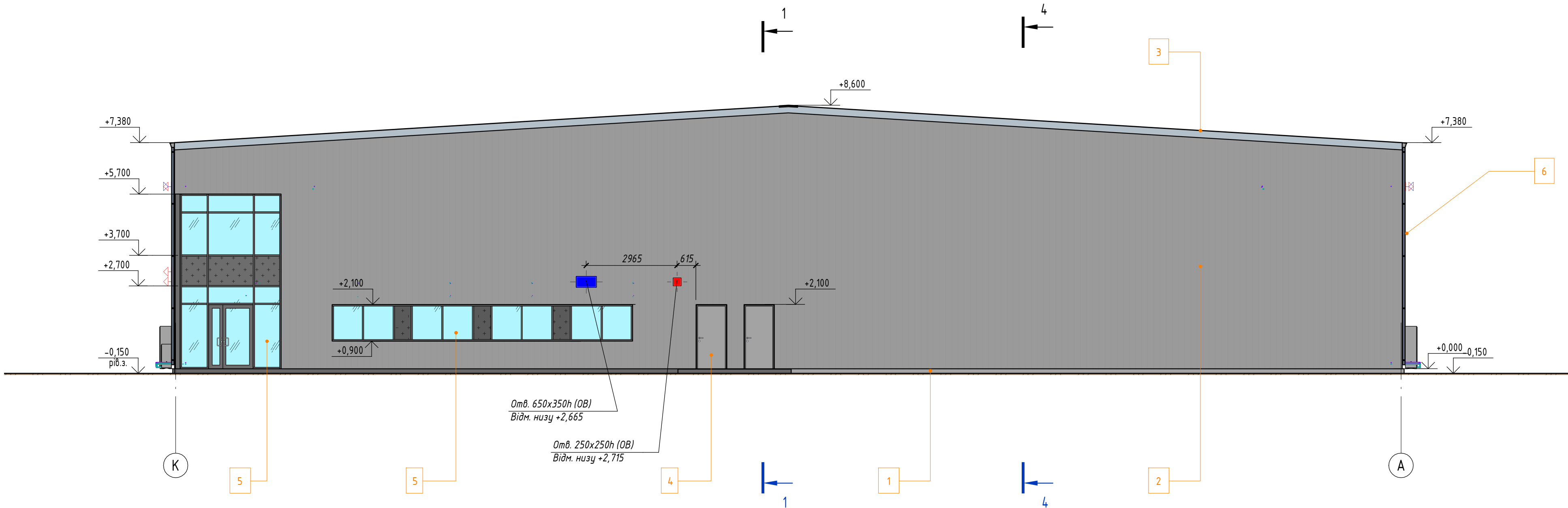
Фасад К - А
