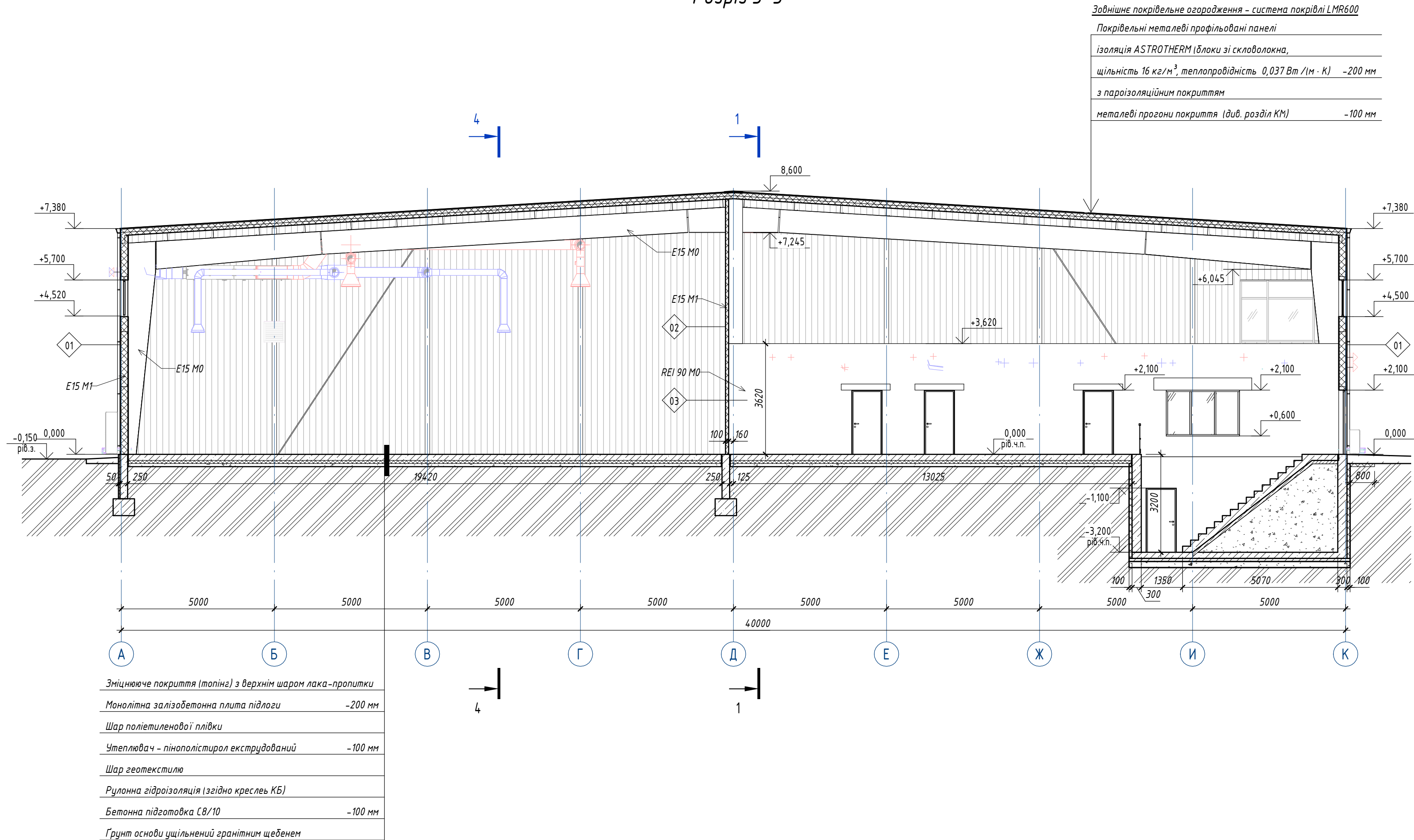
Розріз 3-3
