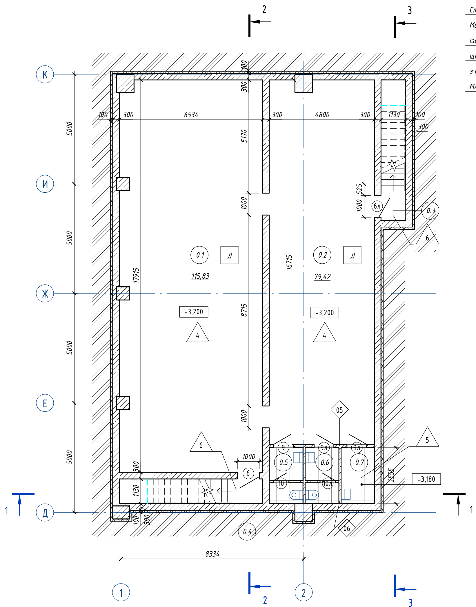
План підвалу
