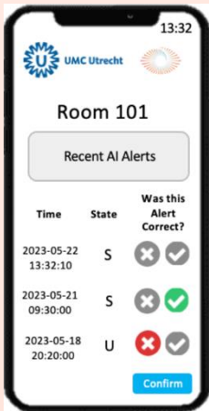
AI Clicker
