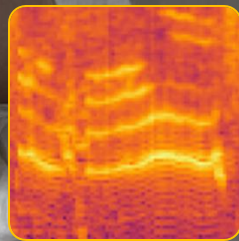
Cry AI
