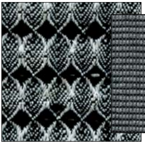
LL544DT (white/black), 313 ± 31 g/m 2 , 100 % linen, width 155 ± 5 cm
