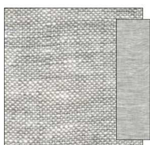
LL519T, 190 ± 20 g/m², 100 % linen, width 230 ± 5 cm
