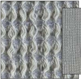
CL461T, 650 ± 65 g/m 2 , 50 % linen 50 % cotton, width 185 ± 5 cm
