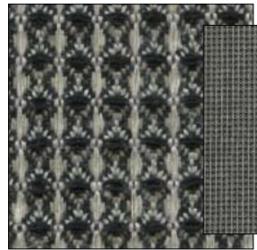
CL922, 320 ± 30 g/m 2 , 50 % linen 50 % cotton, width 155 ± 5 cm
