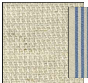
CL382, 210 ± 20 g/m 2 , 50 % linen 50 % cotton, width 50 ± 5 cm
