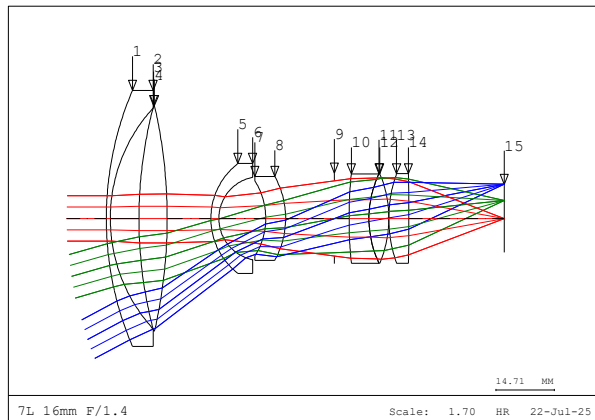
CodeV
