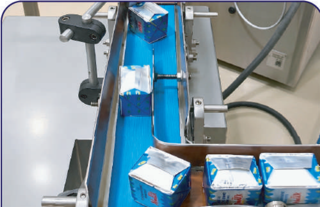
ÜRÜN ÇEVİRME SİSTEMİ PRODUCT INVERTING SYSTEM
