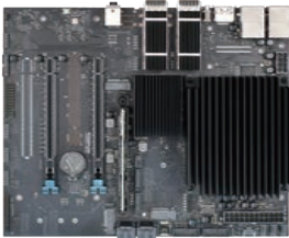
IGX Thor™ T7000 128GB 5581 FP4 TFLOPS
