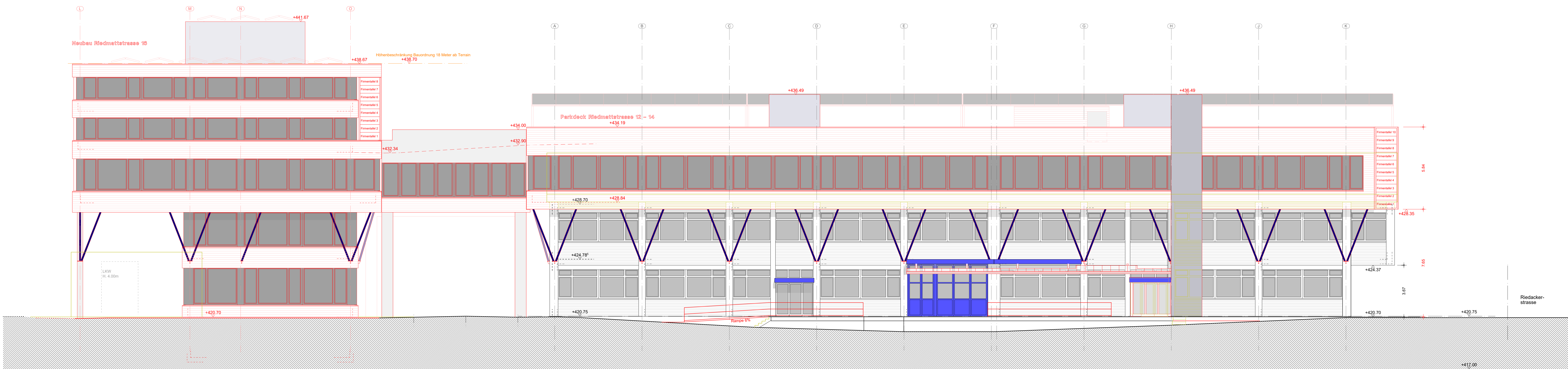
Fassade Süd
