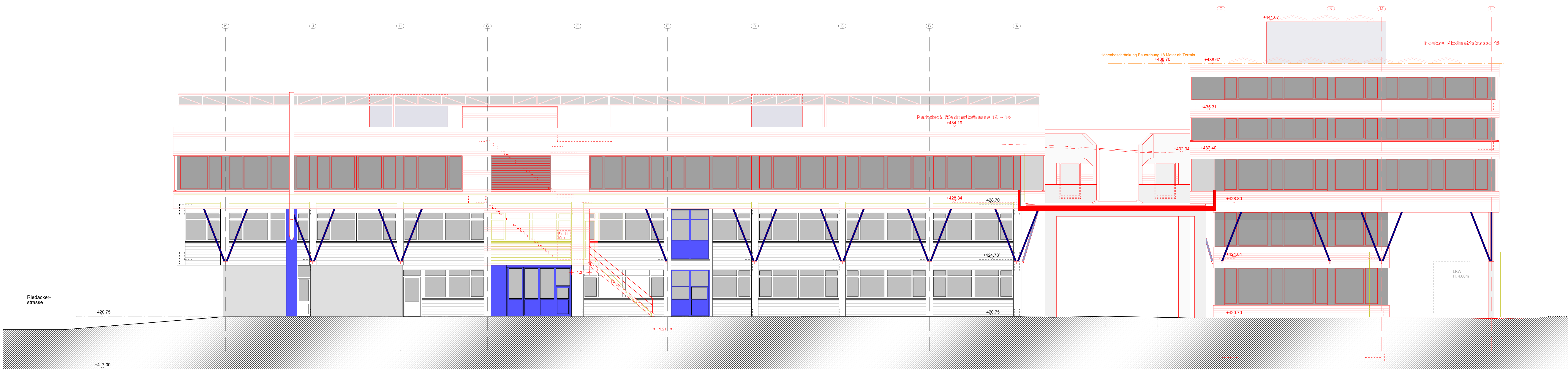
Fassade Nord
