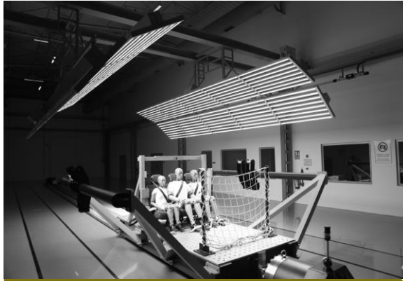
Sled Test
